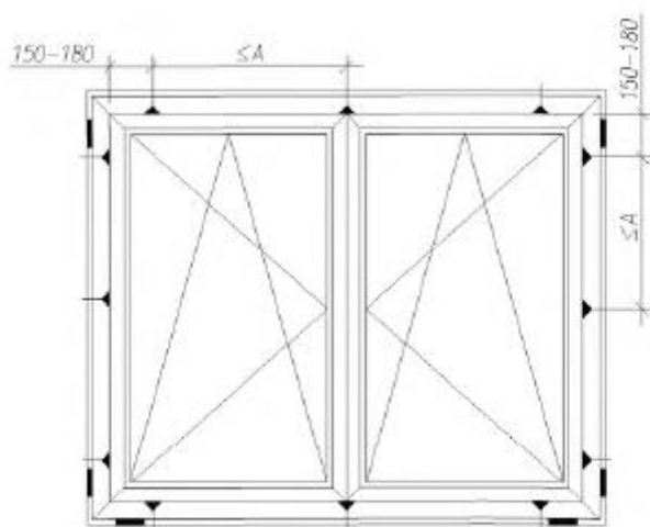
б) Оконный блок с безымпостным (штульповым) притвором
